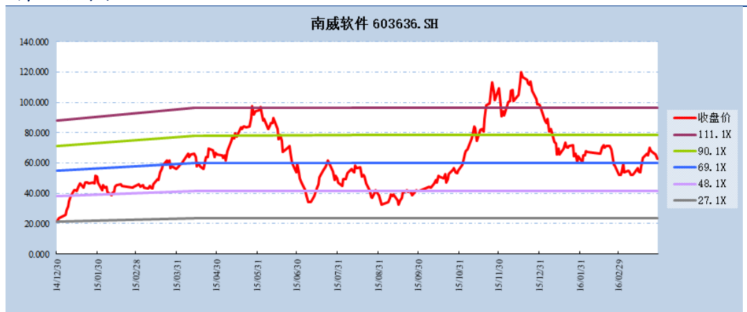
图 3：公司的 PE-Band
